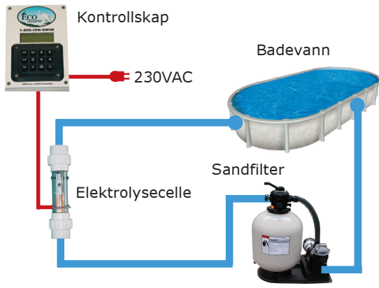
Koblingsskjema - Spa, Standard & Turbo
