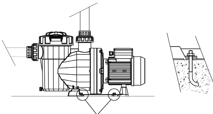
Anchor detail / Detail de l'ancrage Detalle anclaje / Dettaglio ancoraggio Verankerung / Anker detail / Detalhe de fixação Λεπτομέρεια αγκίστρου / تفصيل التثبيت
