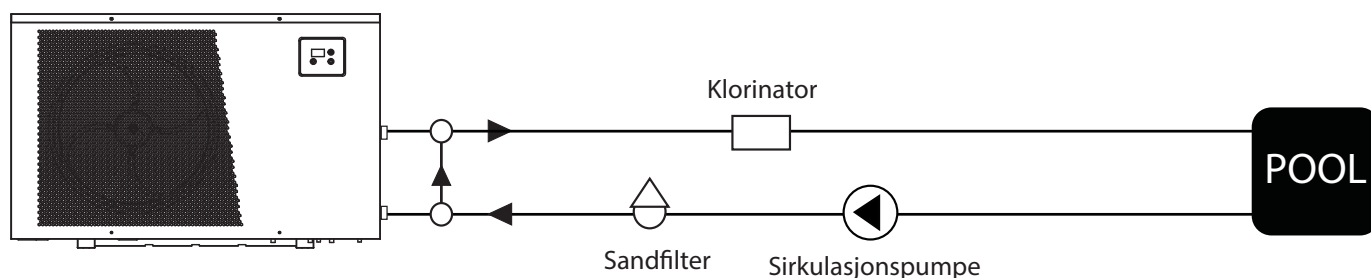
Prinsippskisse for installasjon av X-serien
