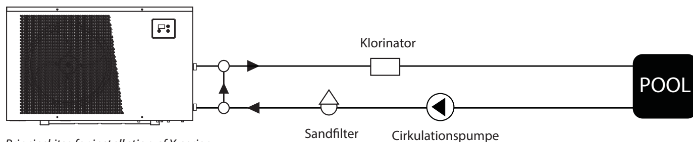
Principskitse for installation af X-serien
