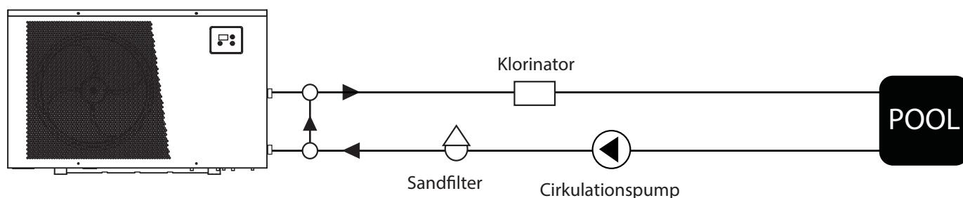
Principskiss för installation av X-serien
